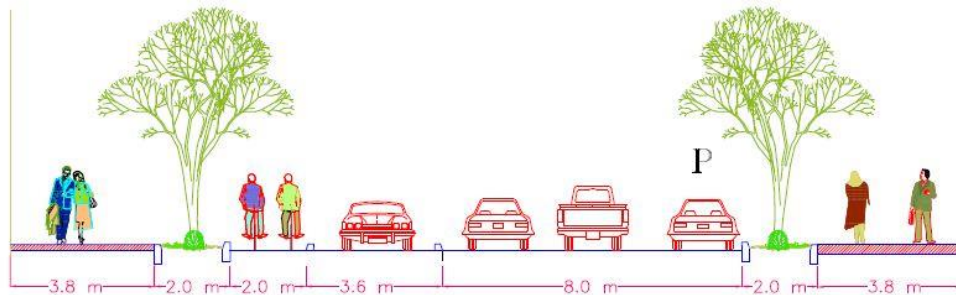
(مقطع مسیر دوچرخه خیابان حافظ)
